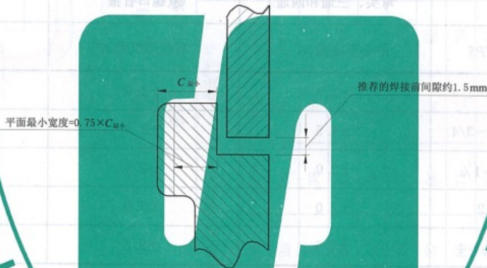
图 6.1.3 要求的焊接间隙和平面最小宽度
