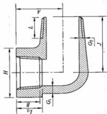
图 4.1.6 内外螺纹 90° 弯头
